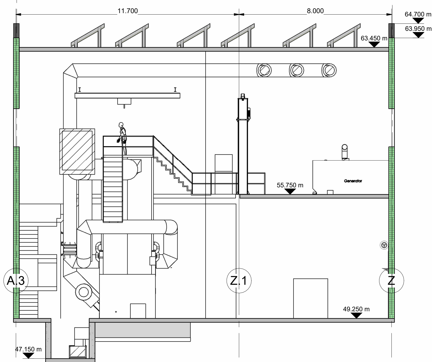
SECTION 2 Scale 1 : 100
