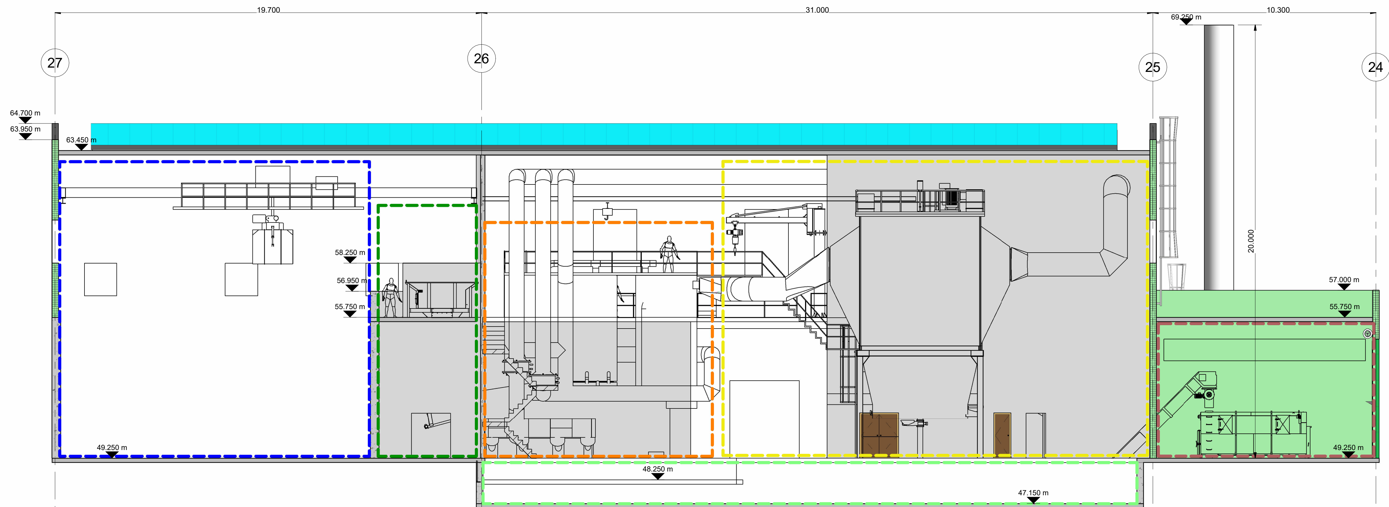
SECTION 1 Scale 1 : 100
